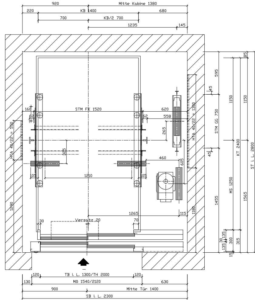
Schachtgrundriß M 1:20
