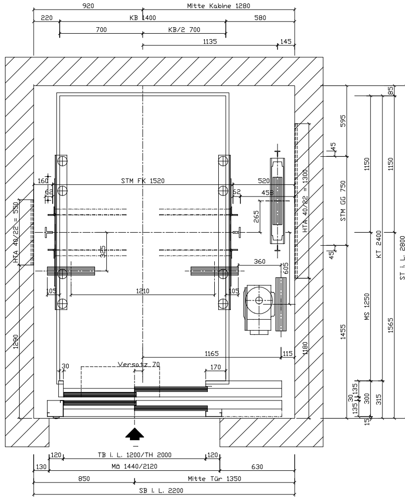
Schachtgrundriß M 1:20
