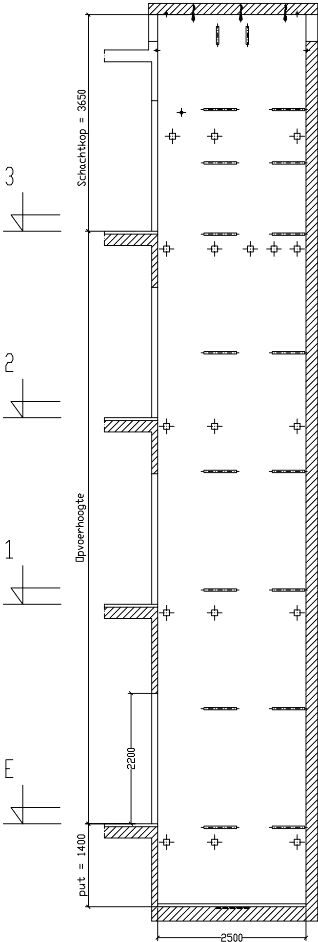
Snijlijn A-A
