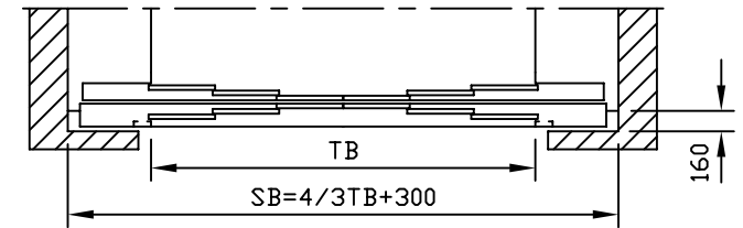
Cabinedeur: 6-dlg. teleskoopschuivdeur centraal Schachtdeur: 6-dlg. teleskoopschuivdeur centraal Montage in metselwerknis
