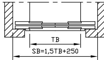
Cabinedeur: 4-dlg. teleskoopschuivdeur centraal Schachtdeur: 4-dlg. teleskoopschuivdeur centraal Montage op schachtwand
