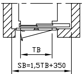
Cabinedeur: 2-dlg. teleskoopschuivdeur eenzijdig Schachtdeur: draaideur met een vleugel, manueel
