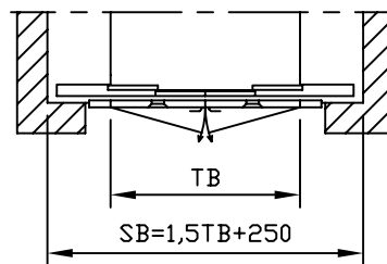
Cabinedeur: 4-dlg. teleskoopschuivdeur centraal Schachtdeur: draaideur met twee vleugel, manueel
