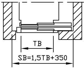
Cabinedeur: 2-dlg. teleskoopschuivdeur eenzijdig Schachtdeur: 2-dlg. teleskoopschuivdeur eenzijdig Montage op schachtwand
