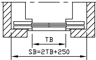
Cabinedeur: 2-dlg. teleskoopschuivdeur centraal Schachtdeur: 2-dlg. teleskoopschuivdeur centraal Montage op schachtwand
