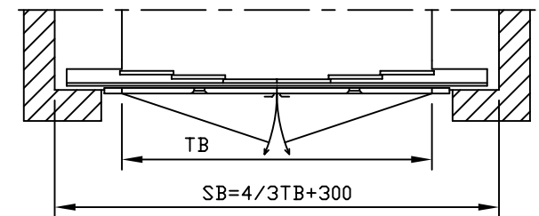
Cabinedeur: 6-dlg. teleskoopschuivdeur centraal Schachtdeur: draaideur met twee vleugel, manueel
