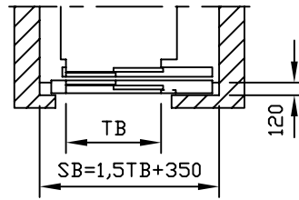
Cabinedeur: 2-dlg. teleskoopschuivdeur eenzijdig Schachtdeur: 2-dlg. teleskoopschuivdeur eenzijdig Montage in metselwerknis
