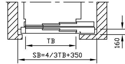
Cabinedeur: 3-dlg. teleskoopschuivdeur eenzijdig Schachtdeur: 3-dlg. teleskoopschuivdeur eenzijdig Montage in metselwerknis
