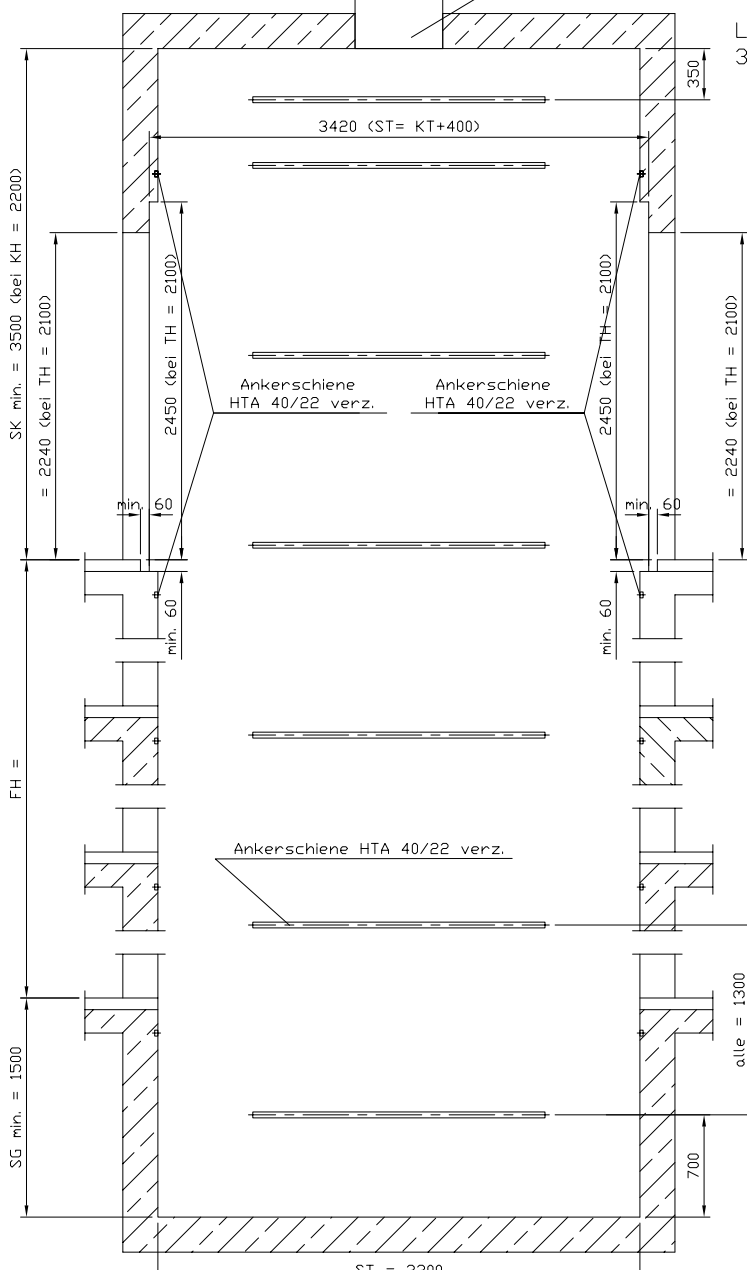
Schnitt A-A 1500
