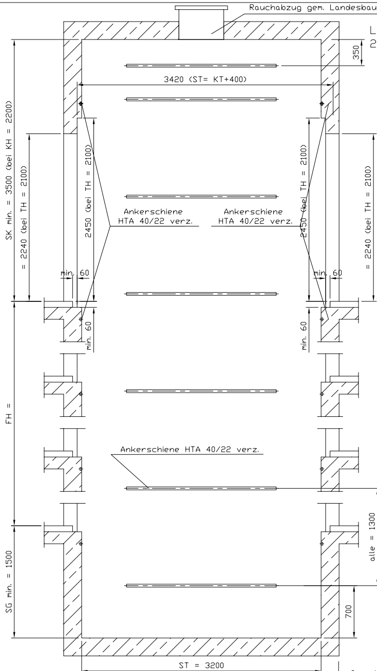
Schnitt A-A
