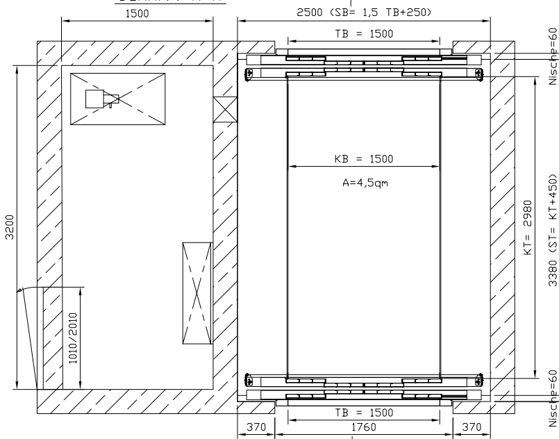
Schnitt A-A
